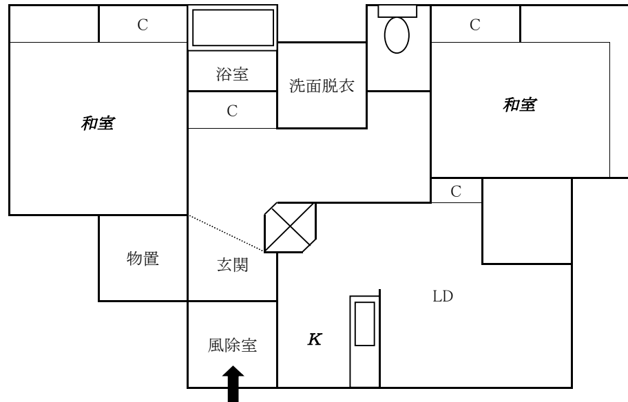
—1階平面図—
